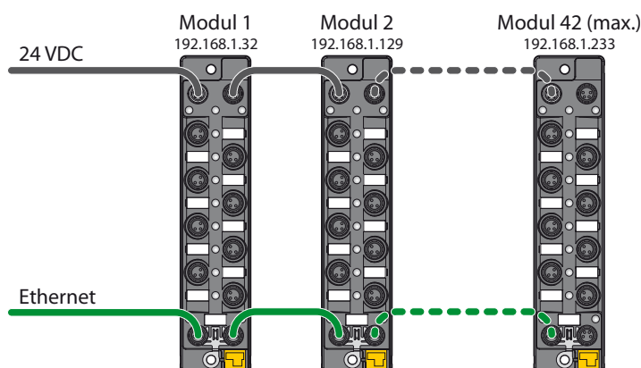
Fig. 83: Daisy Chain
